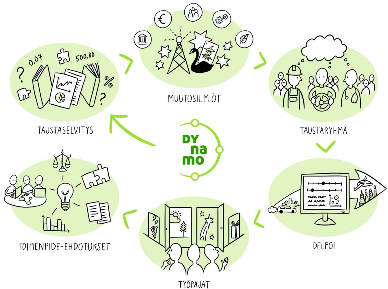
Kuva 1. Dynamo-prosessi
